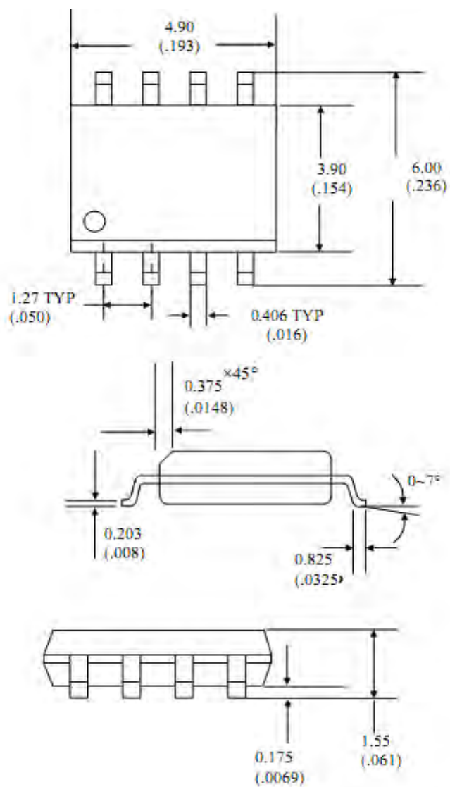
SOP8L 外形图
