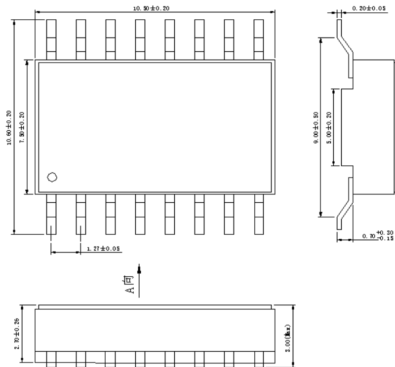
CSOP16D 外形图
