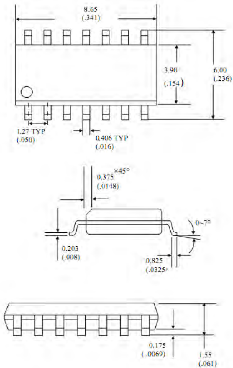
SOP14L 外形图
