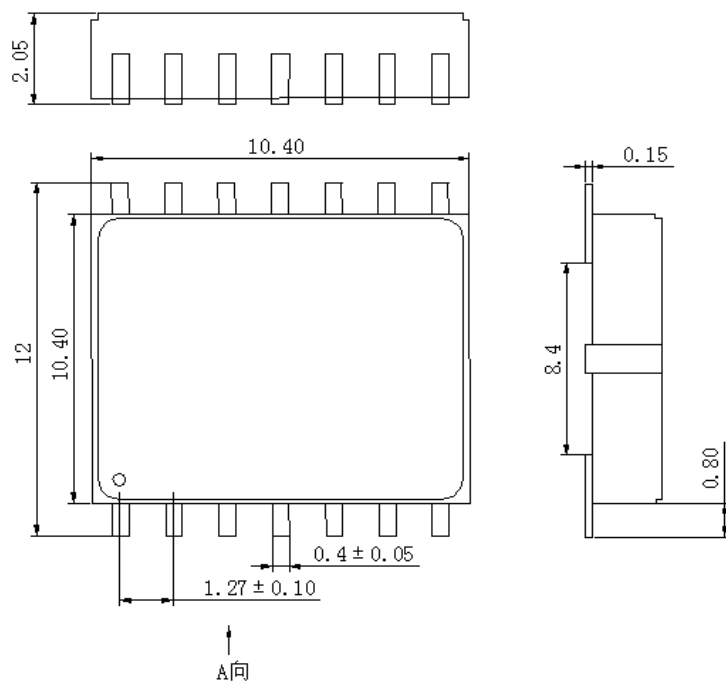
F14-03外形图
