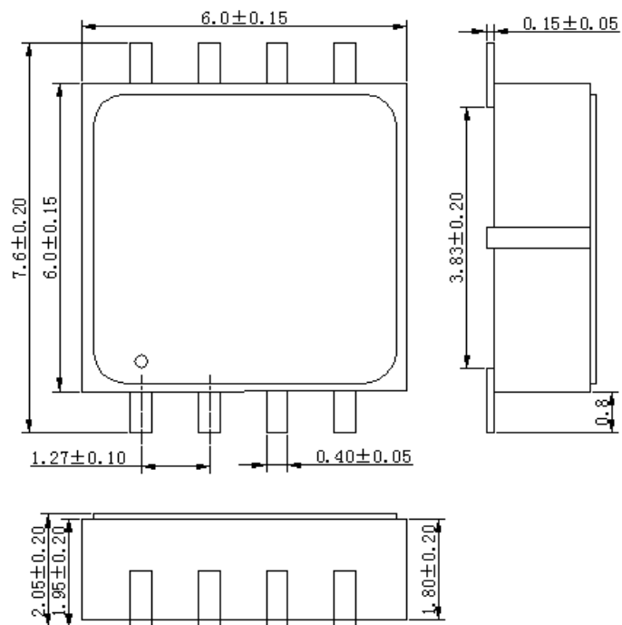
F08-06 外形图
