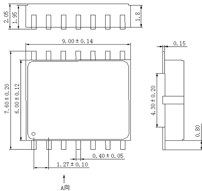
F14-01外形图
