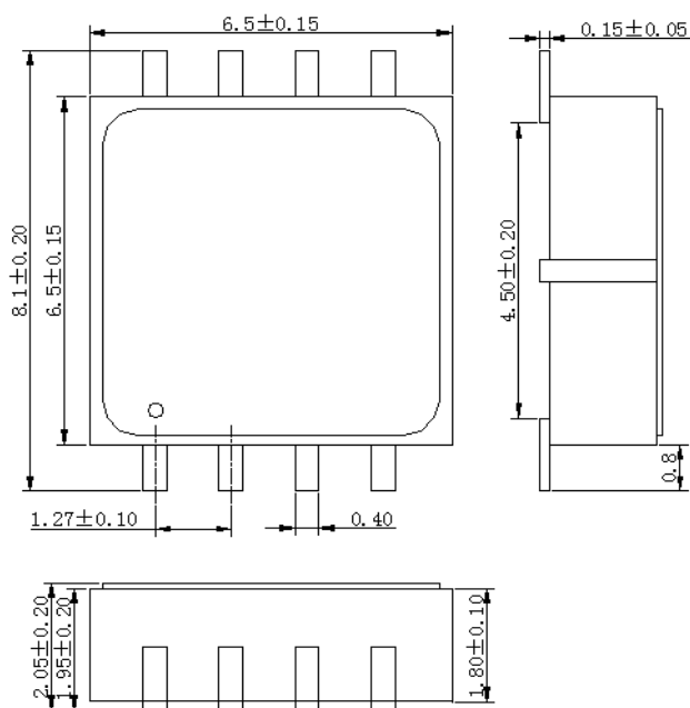
F08-04外形图
