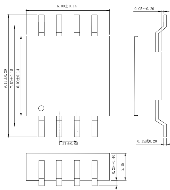
CSOP08 外形图
