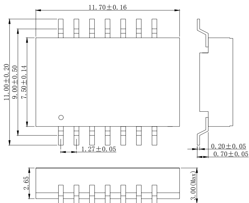
CSOP14 外形图
