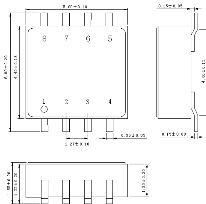
CSOP08B 外形图
