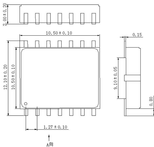
FP14D外形图
