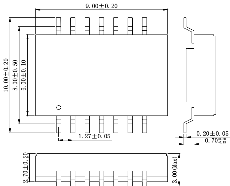
CSOP14B 外形图
