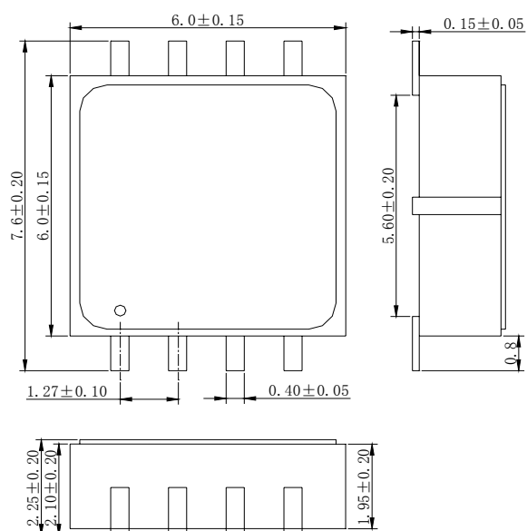
F08-02 外形图
